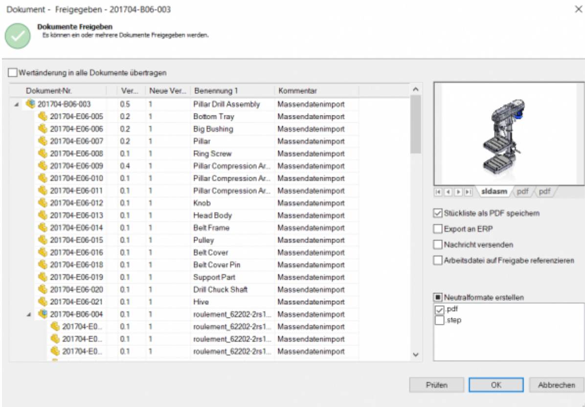
Freigabedialog
