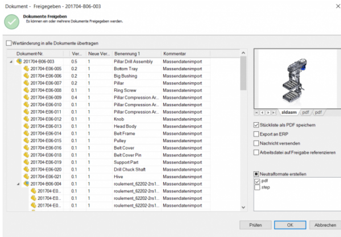
Freigabedialog
