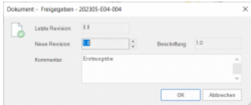
Einfacher Freigabedialog
